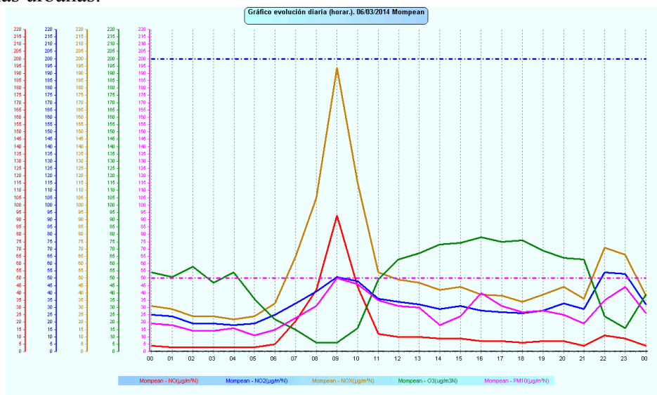
Gráfica 2.- Evolución diaria-horaria del día 06/03/2014 en la estación de inmisión de Mompean para los contaminantes óxidos de nitrógeno, ozono y partículas. Tipo: Urbana de Fondo
