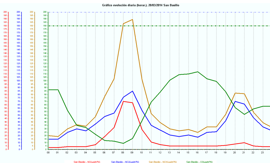
Gráfico 1.- Evolución diaria-horaria del día 20/03/14 en la estación de inmisión de San Basilio para los contaminantes óxidos de nitrógeno y ozono. Tipo: Suburbana de tráfico
